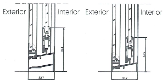
Sección Inferior Sillar Cámara
